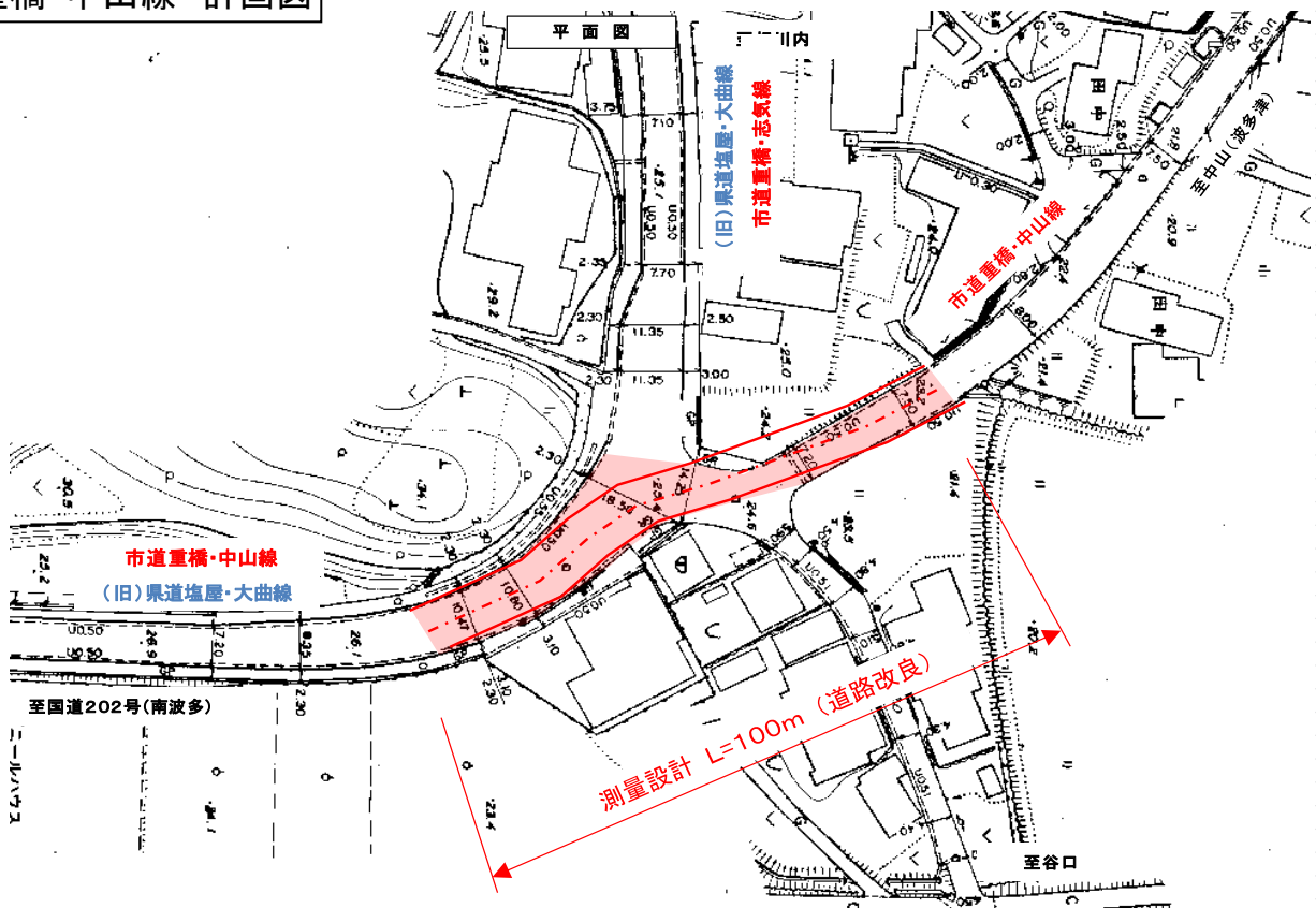
重橋・中山線 計画図
