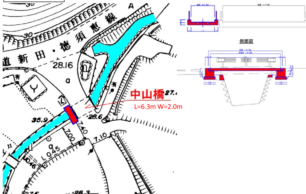
中山橋 計画図
