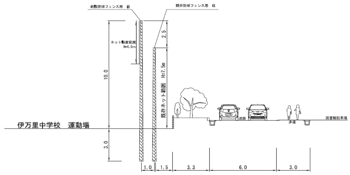
伊万里中学校 防球ネット 断面図
