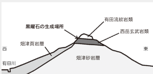
↑腰岳の地質構造(模式図)
