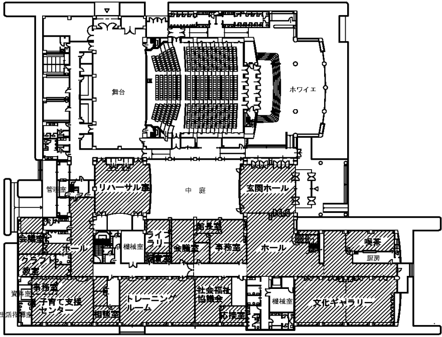
2階改修平面図
