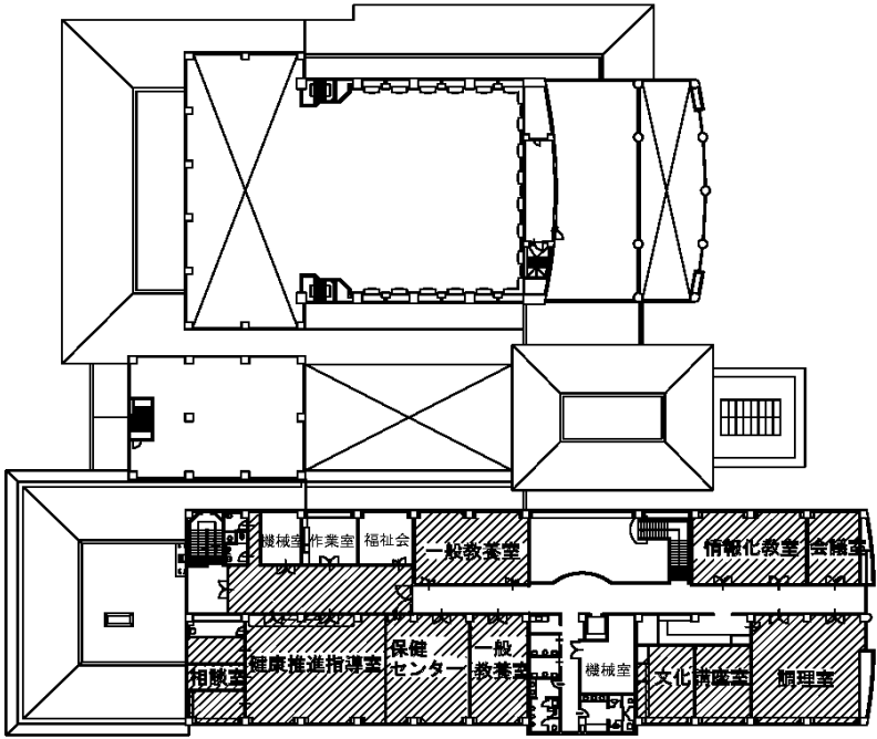
2階改修平面図
