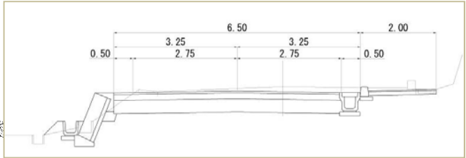
標準断面図
