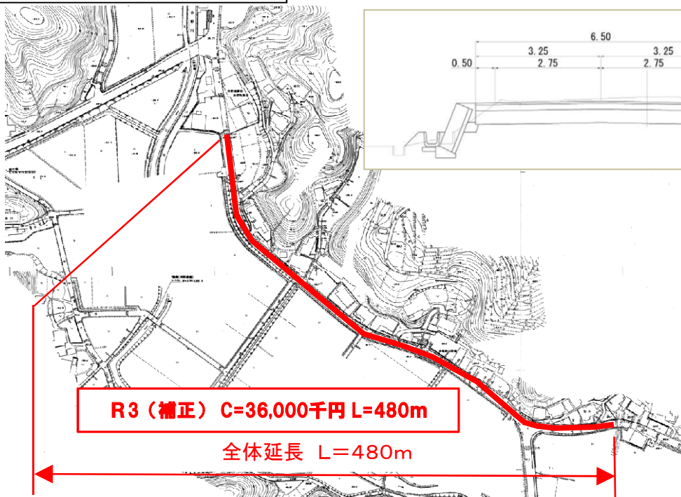
中山・井野尾線 計画図
