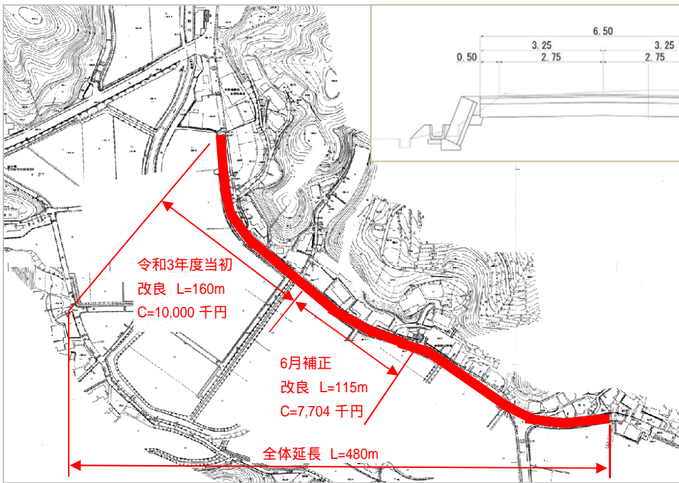
中山・井野尾線 計画図
