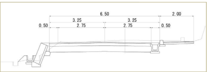
標準断面図
