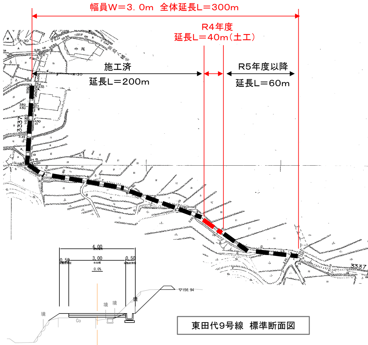
東田代9号線 計画平面図
