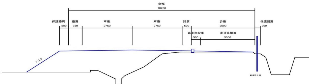
提川・川西線 標準断面図
