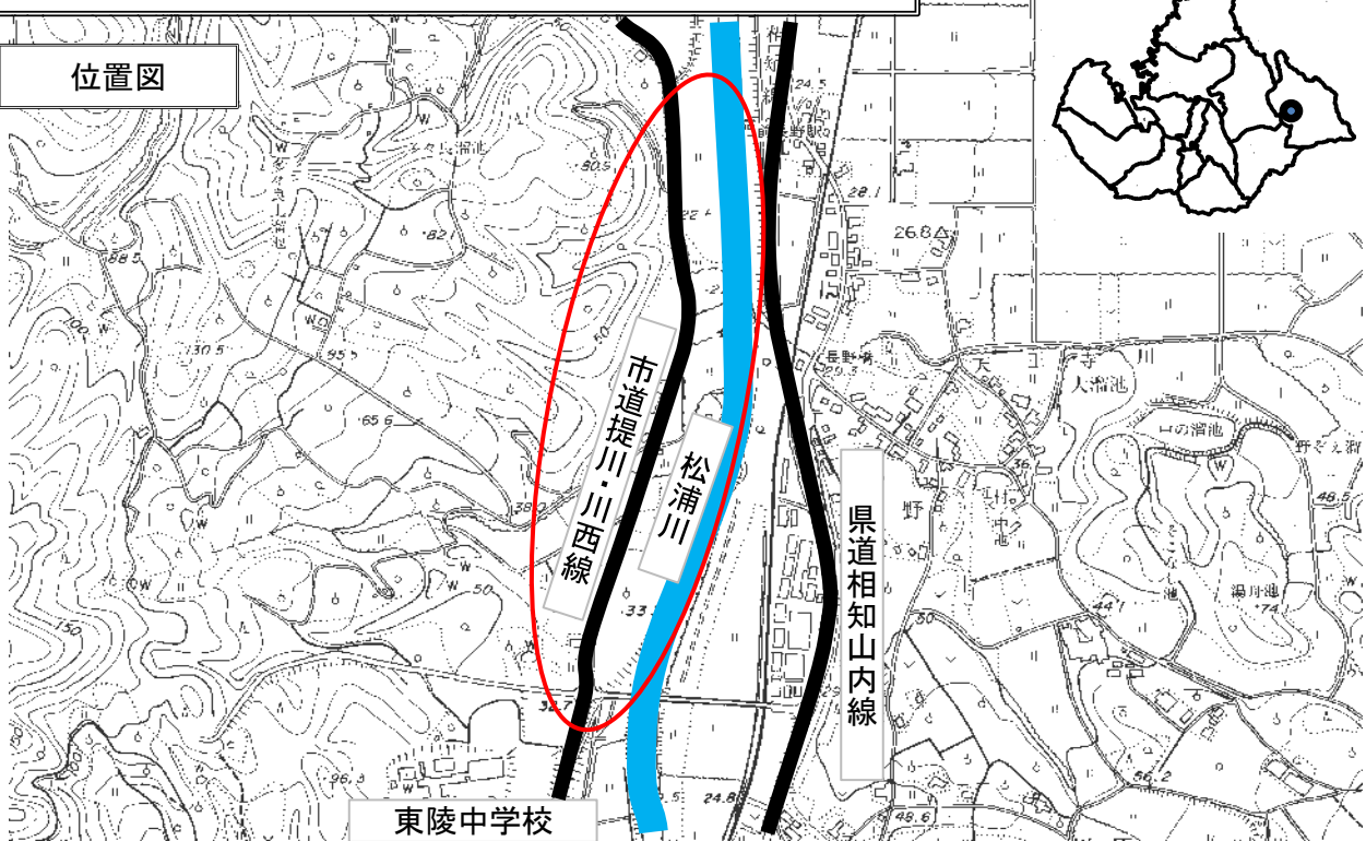
提川・川西線 計画平面図
