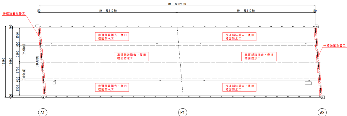
橋面図 s=1:200
