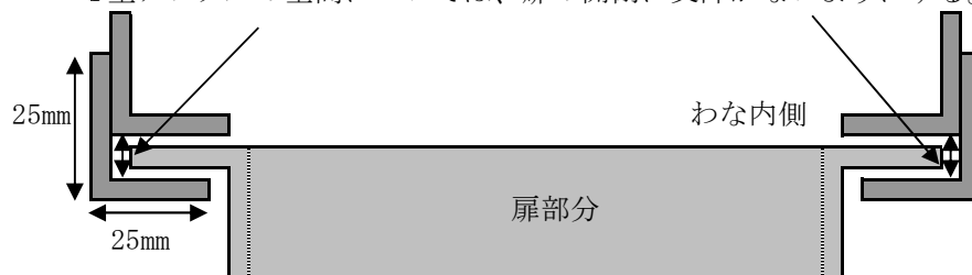
◎レール部分の断面図（真上から）
