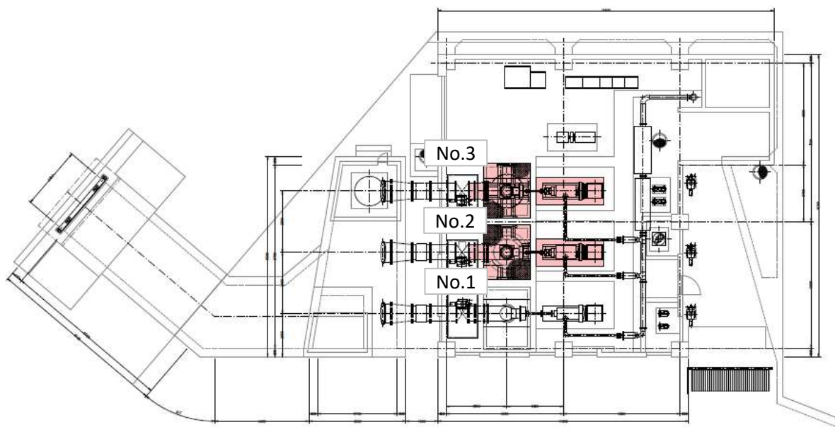
松島雨水ポンプ場 平面図
