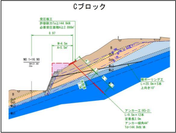
計画断面図
