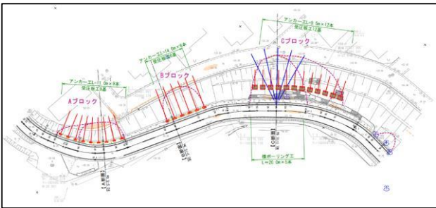
計画平面図
