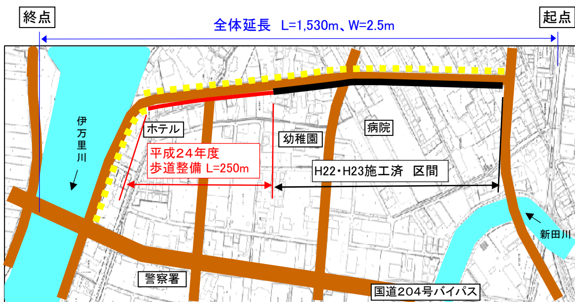
市道八谷搦海岸通り線 計画図
