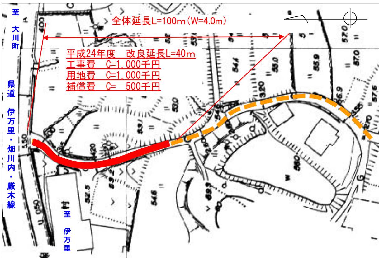
市道笠椎8号線 計画図
