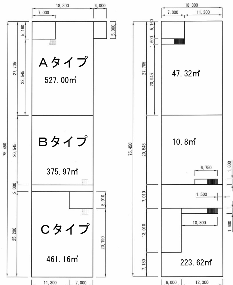
1階平面図
