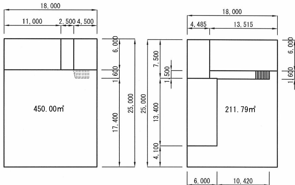
1階平面図
