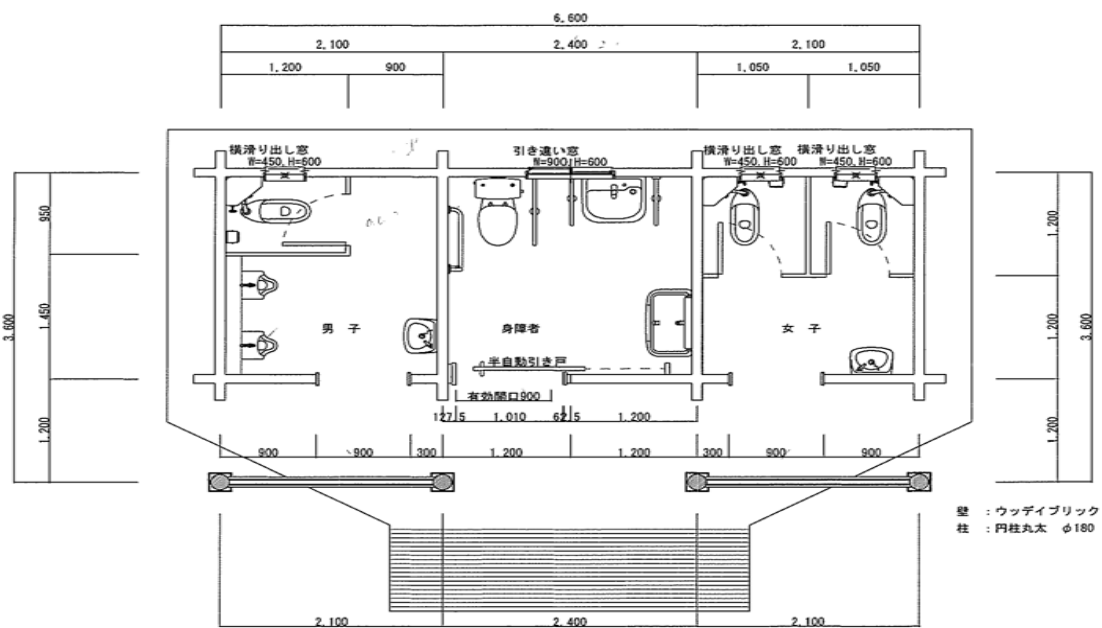
トイレ(D・Eゾーン) 平面図
