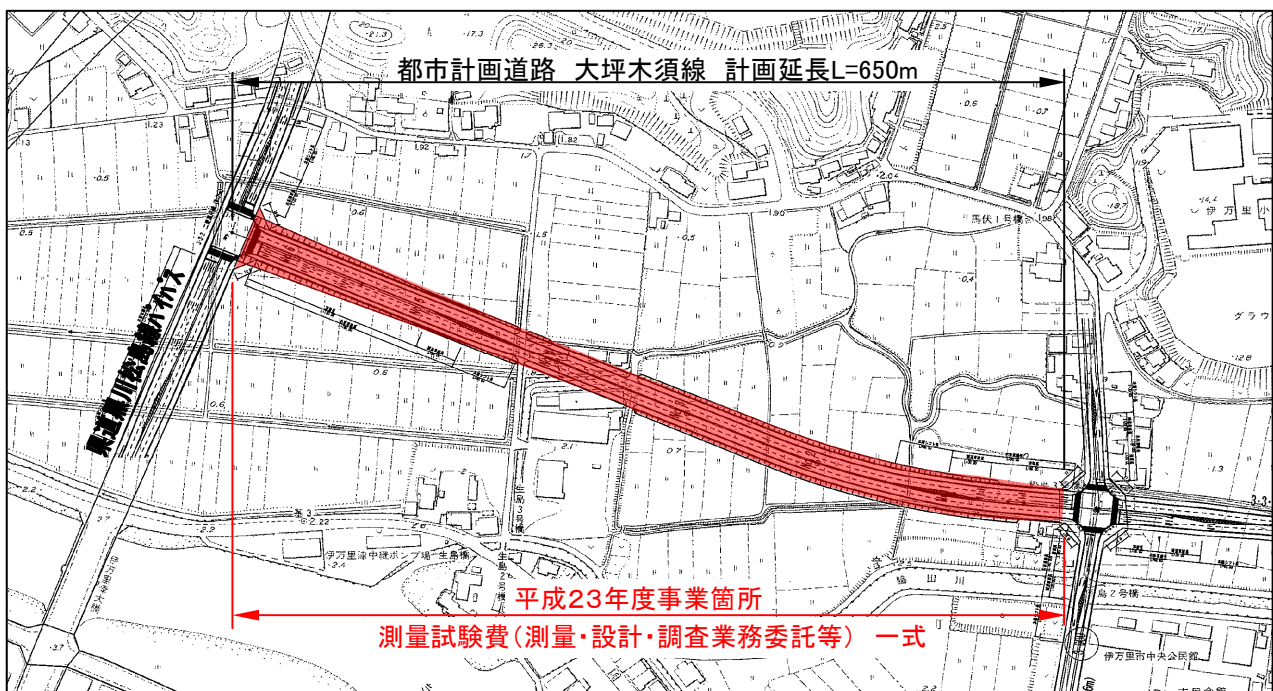
大坪木須線 計画図
