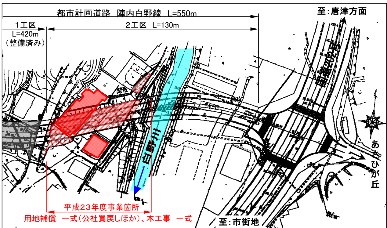
陣内白野線 計画図
