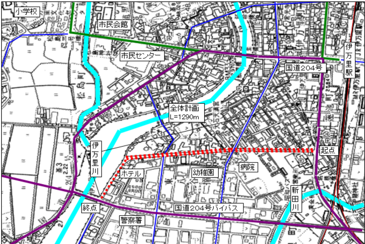
市道八谷搦海岸通り線 位置図
