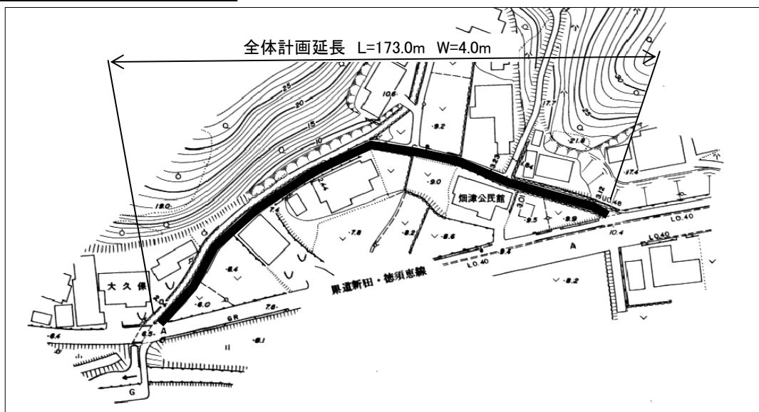
市道畑津4号線 計画図
