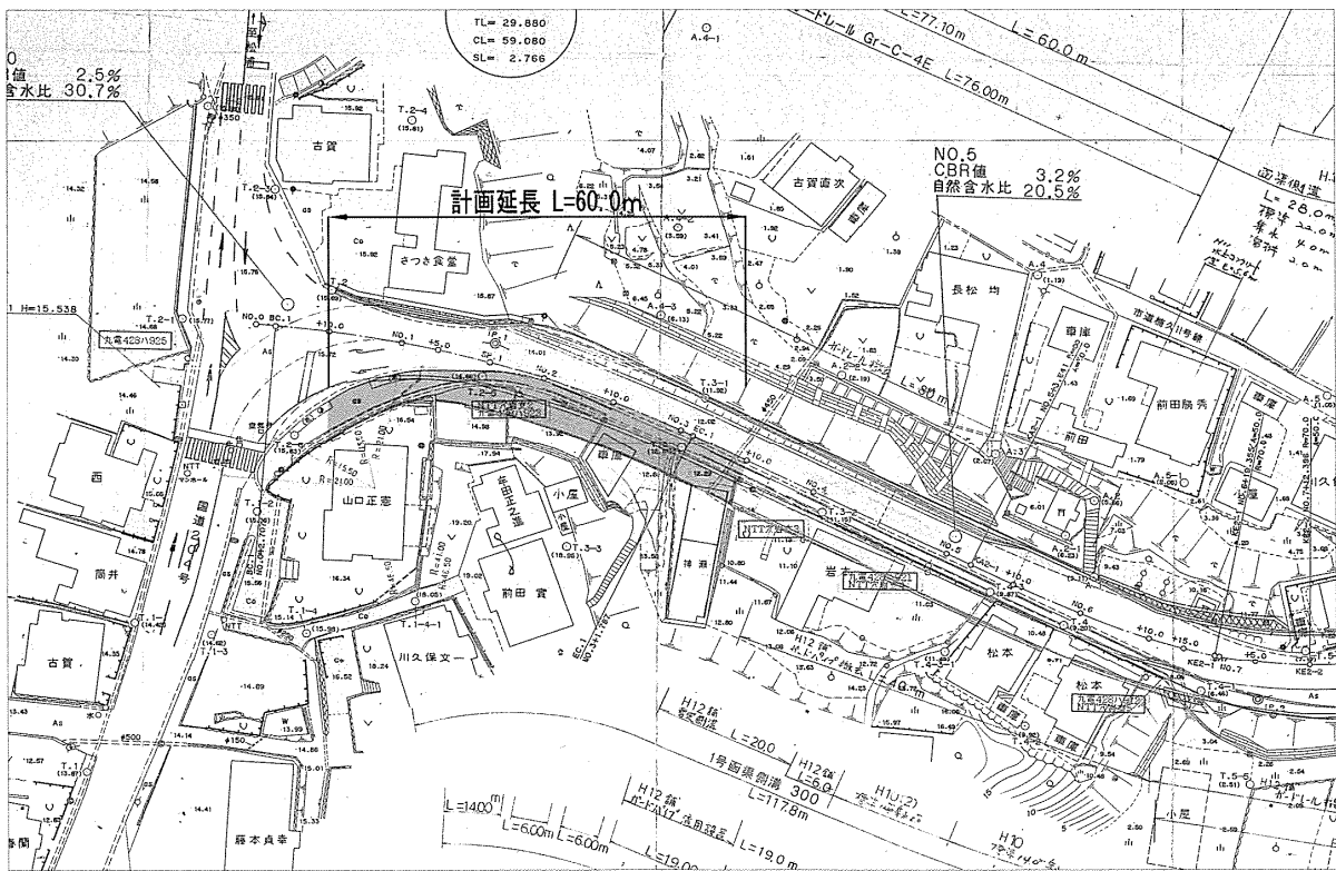
市道四軒屋・福川内・鳴石線 計画図
