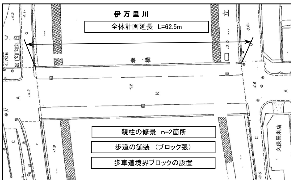
幸橋 計画図
