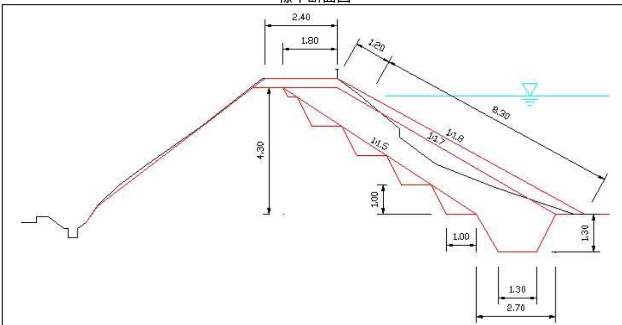
標準断面図
