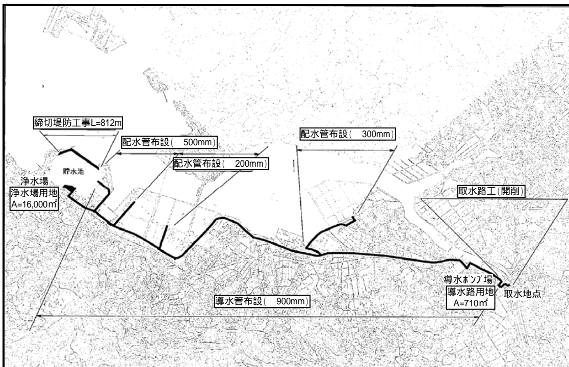
全体計画図
