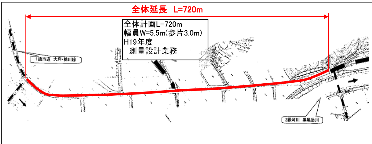
計画図
