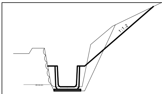
標準断面図
