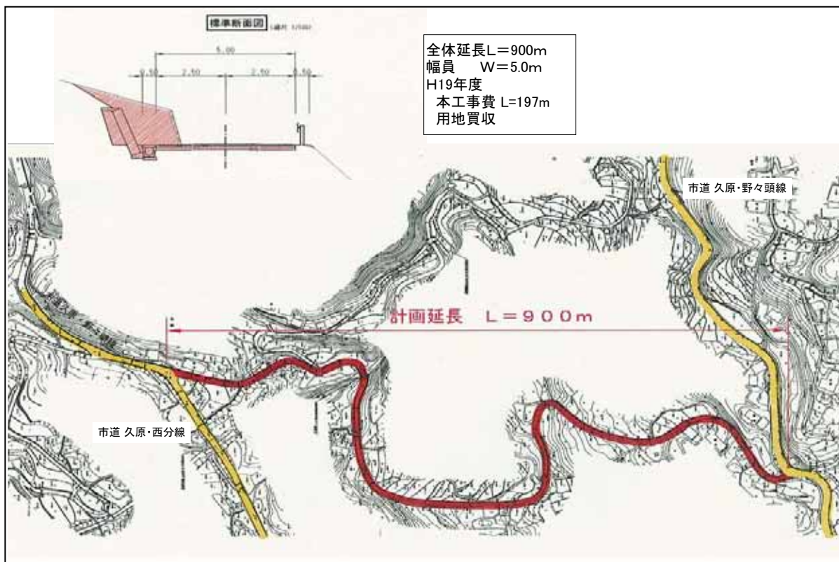
計画図
