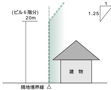
隣地斜線説明図
