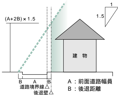
道路斜線説明図
