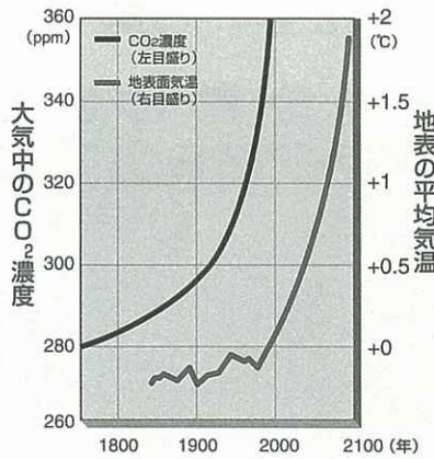
CO 2 濃度と気温の関係 (将来予測値を含む)
